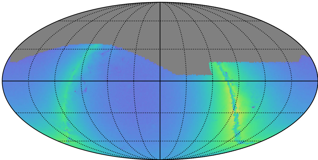
weather_cloudso4v3.4_10yrs g: Nstars_no_crowding
