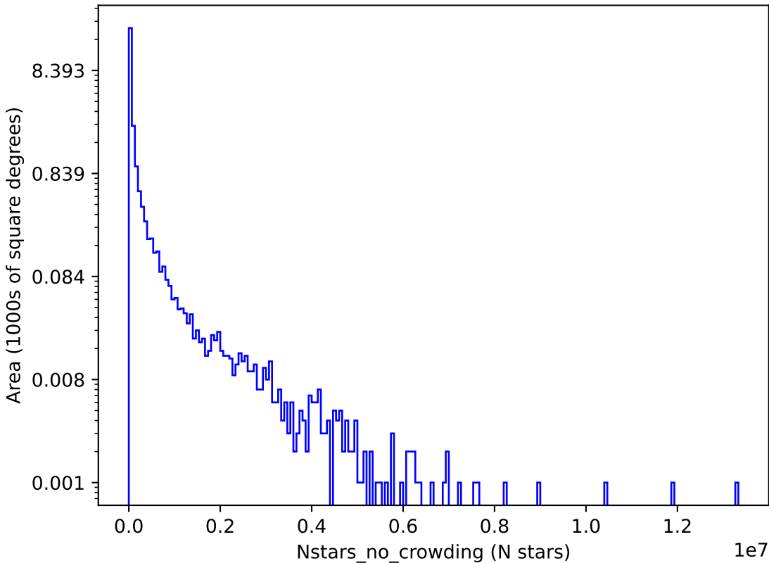
weather_cloudso4v3.4_10yrs g: Nstars_no_crowding
