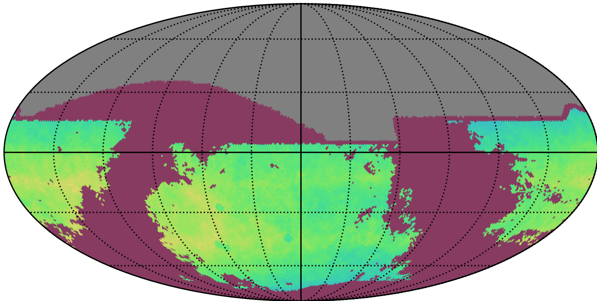
weather_cloudso4v3.4_10yrs i: NgalScale
