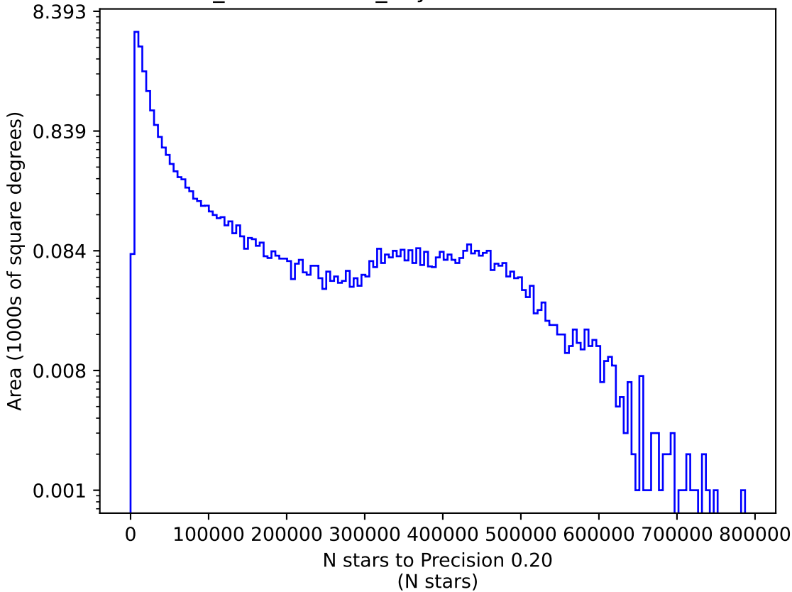
weather_cloudso4v3.4_10yrs i: N stars to Precision 0.20
