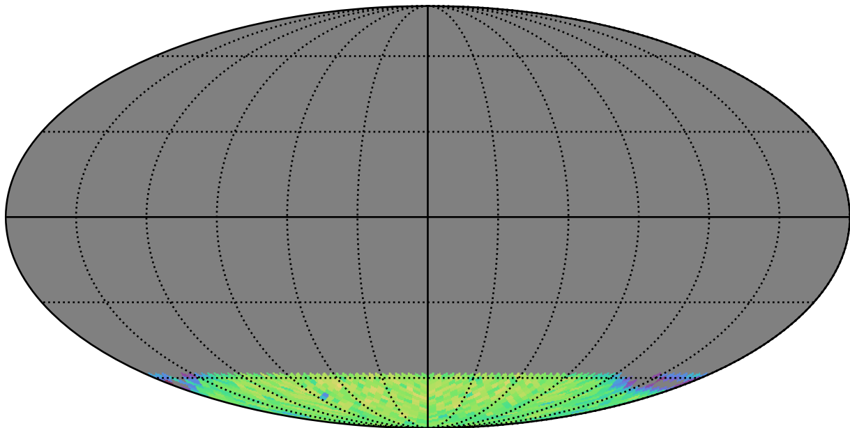
weather_cloudso4v3.4_10yrs gi SCP: LVDwarfs
