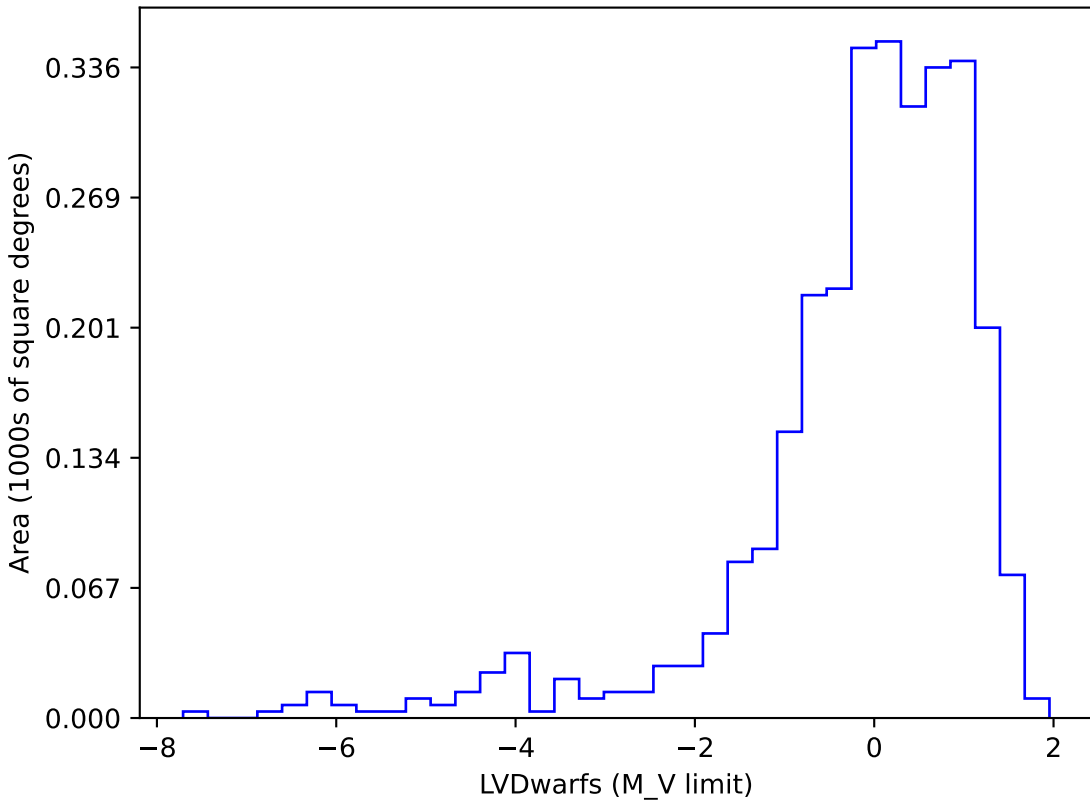
weather_cloudso4v3.4_10yrs gi SCP: LVDwarfs
