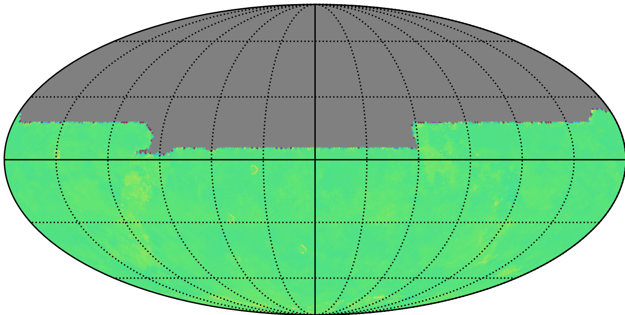
weather_cloudso4v3.4_10yrs y: Kuiper rotTelPos
