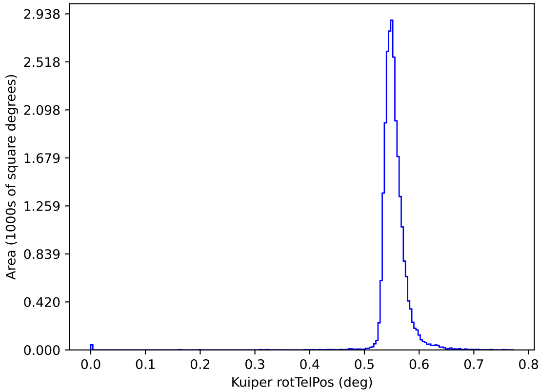
weather_cloudso4v3.4_10yrs y: Kuiper rotTelPos
