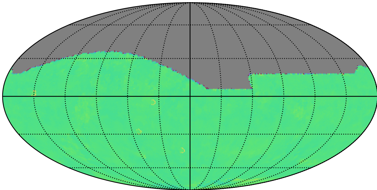
weather_cloudso4v3.4_10yrs r: Kuiper rotTelPos
