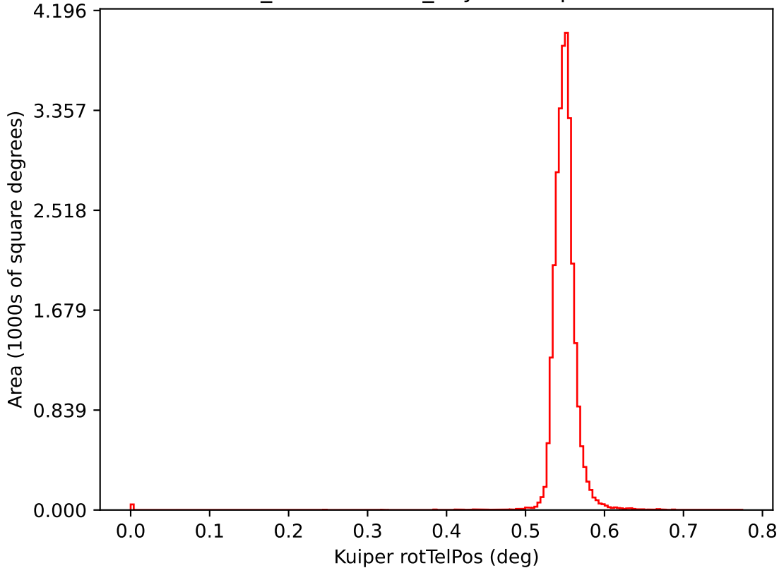
weather_cloudso4v3.4_10yrs i: Kuiper rotTelPos
