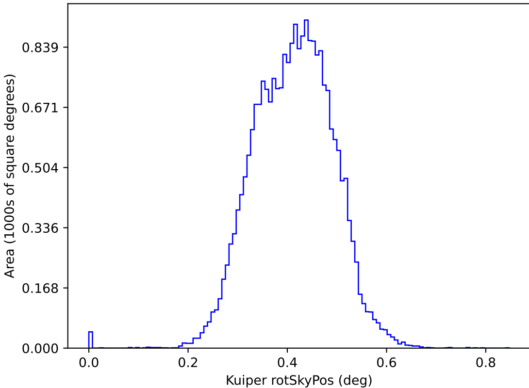
weather_cloudso4v3.4_10yrs y: Kuiper rotSkyPos
