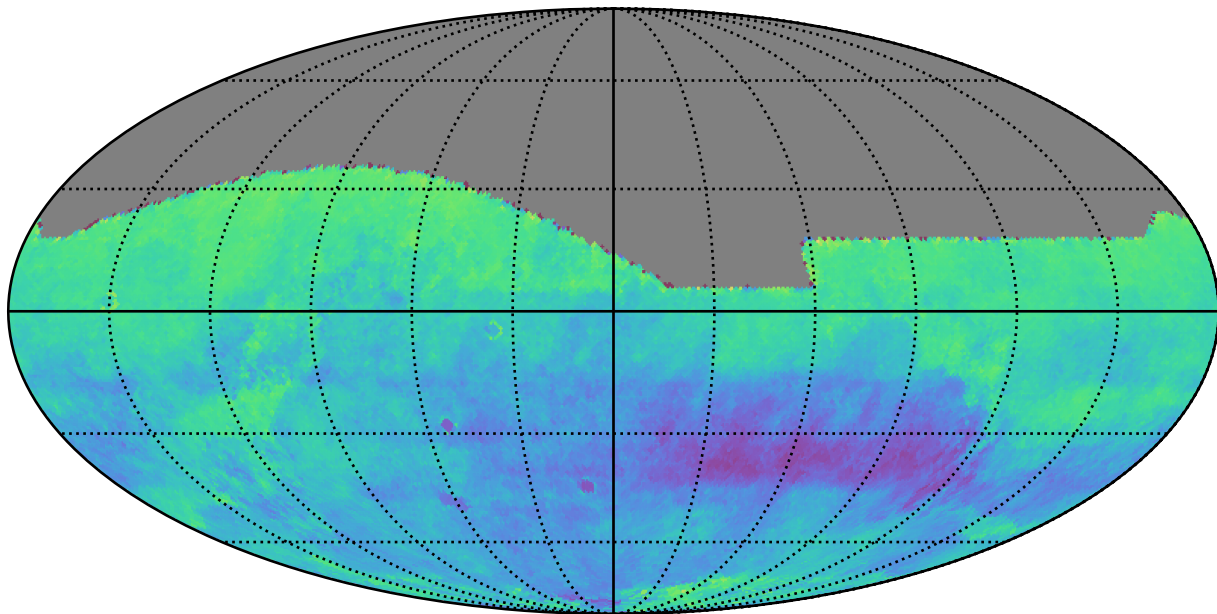
weather_cloudso4v3.4_10yrs r: Kuiper rotSkyPos
