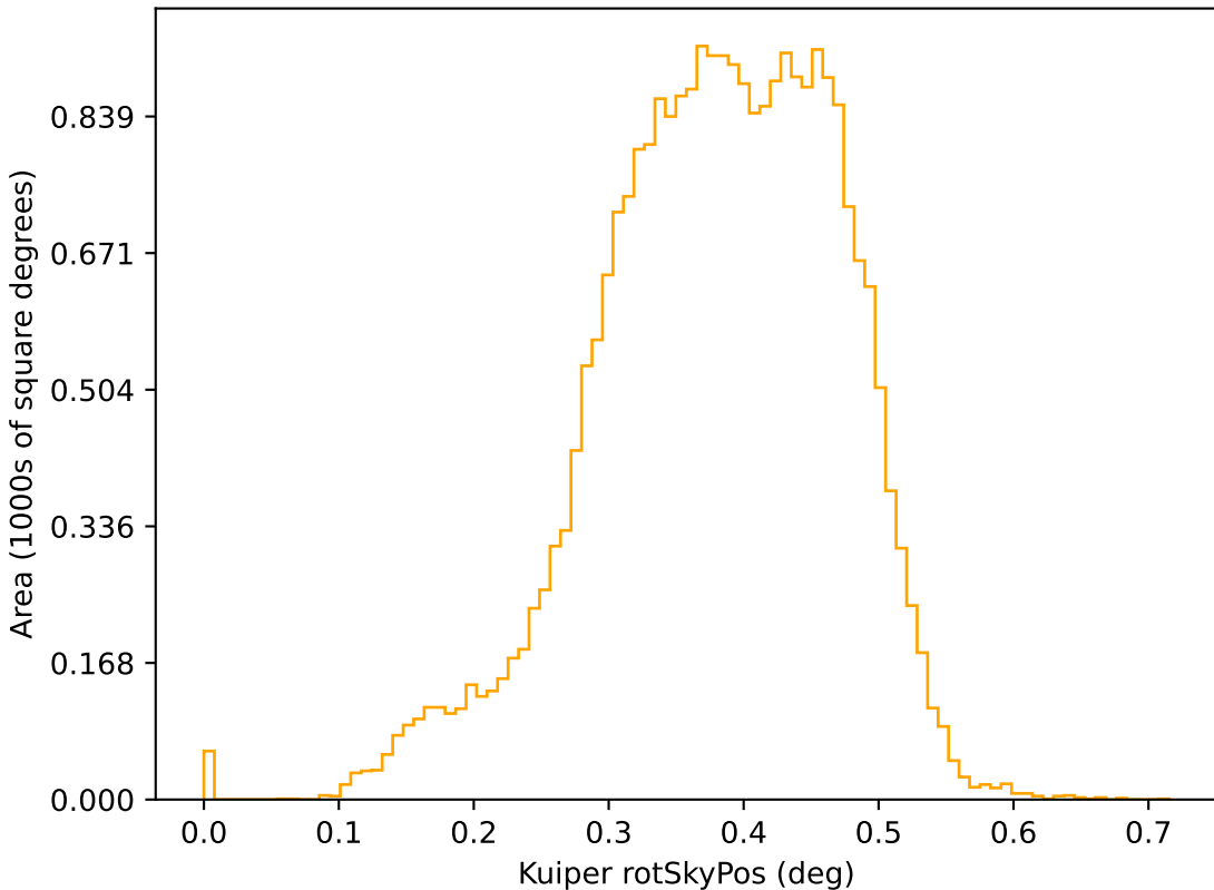
weather_cloudso4v3.4_10yrs r: Kuiper rotSkyPos
