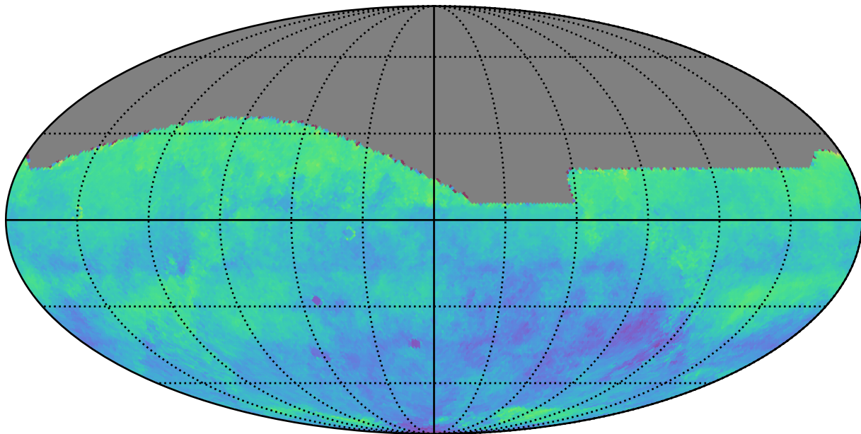
weather_cloudso4v3.4_10yrs i: Kuiper rotSkyPos
