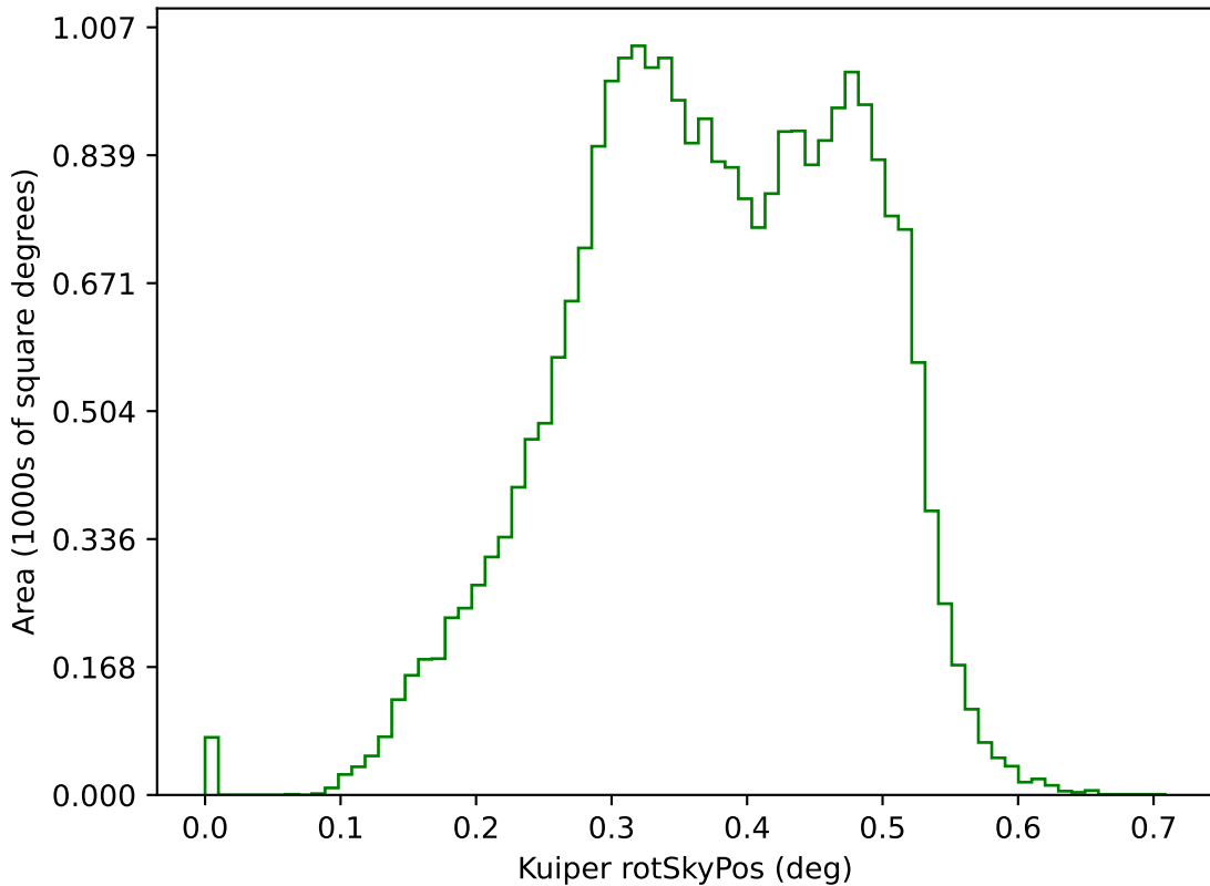
weather_cloudso4v3.4_10yrs g: Kuiper rotSkyPos
