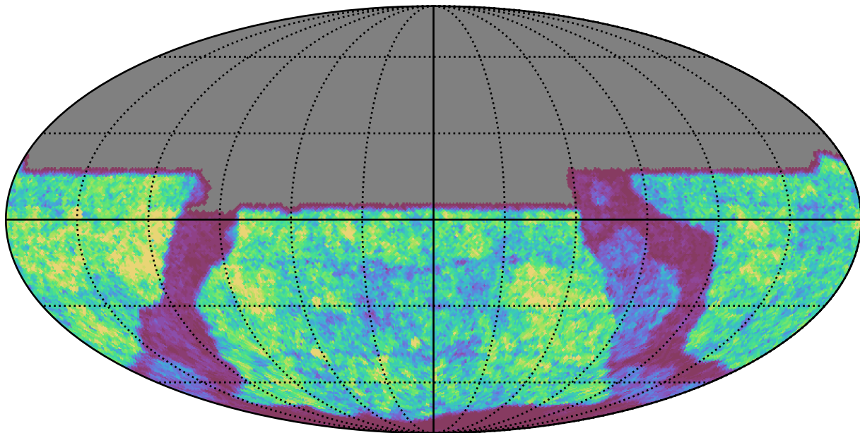
weather_cloudso4v3.4_10yrs y band: Gaps_24hr
