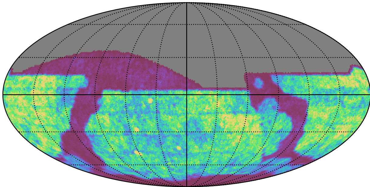
weather_cloudso4v3.4_10yrs i band: Gaps_24hr
