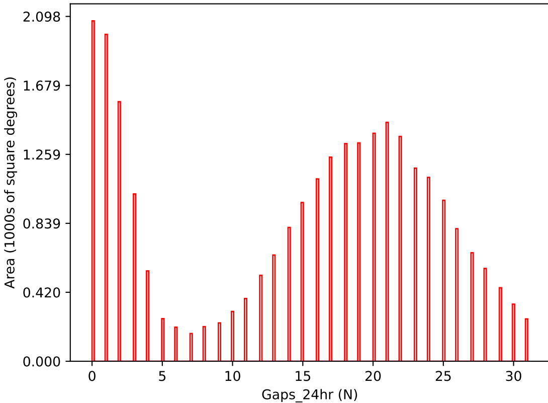
weather_cloudso4v3.4_10yrs i band: Gaps_24hr
