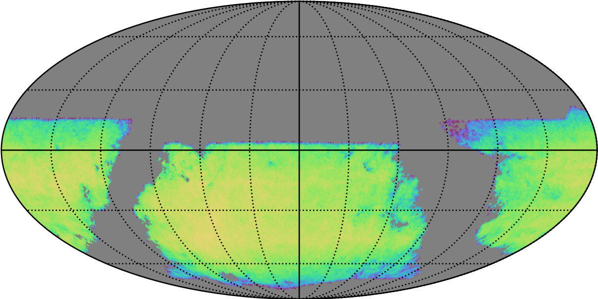
weather_cloudso4v3.4_10yrs i band galaxies non-DD: DepthLimitedNumGalaxiesMetric
