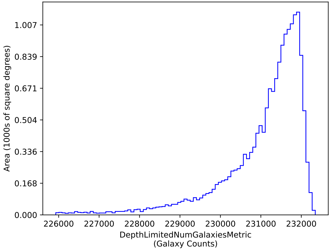
weather_cloudso4v3.4_10yrs i band galaxies non-DD: DepthLimitedNumGalaxiesMetric
