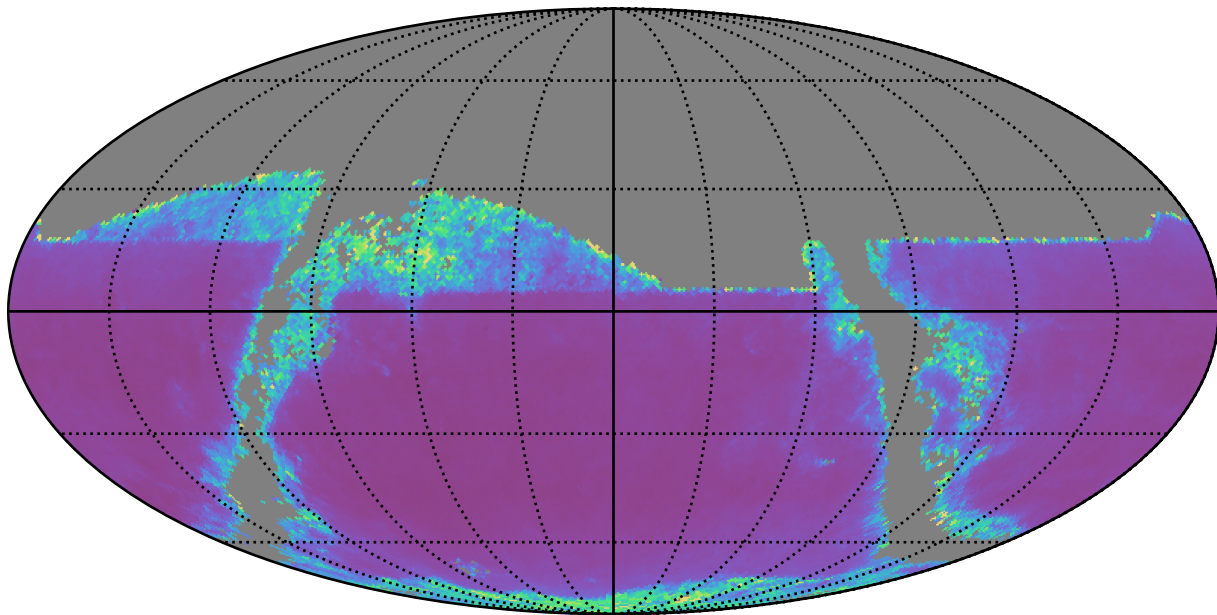
weather_cloudso4v3.4_10yrs z band: AGN SF_uncert
