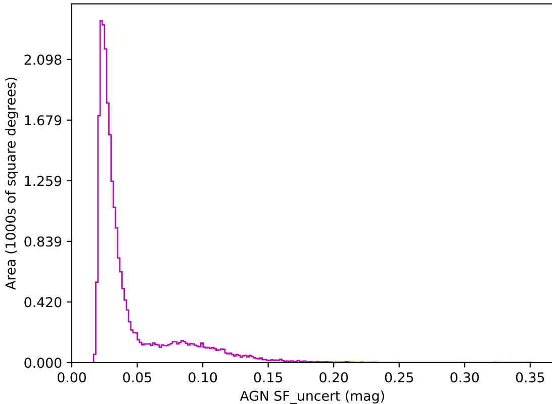
weather_cloudso4v3.4_10yrs z band: AGN SF_uncert
