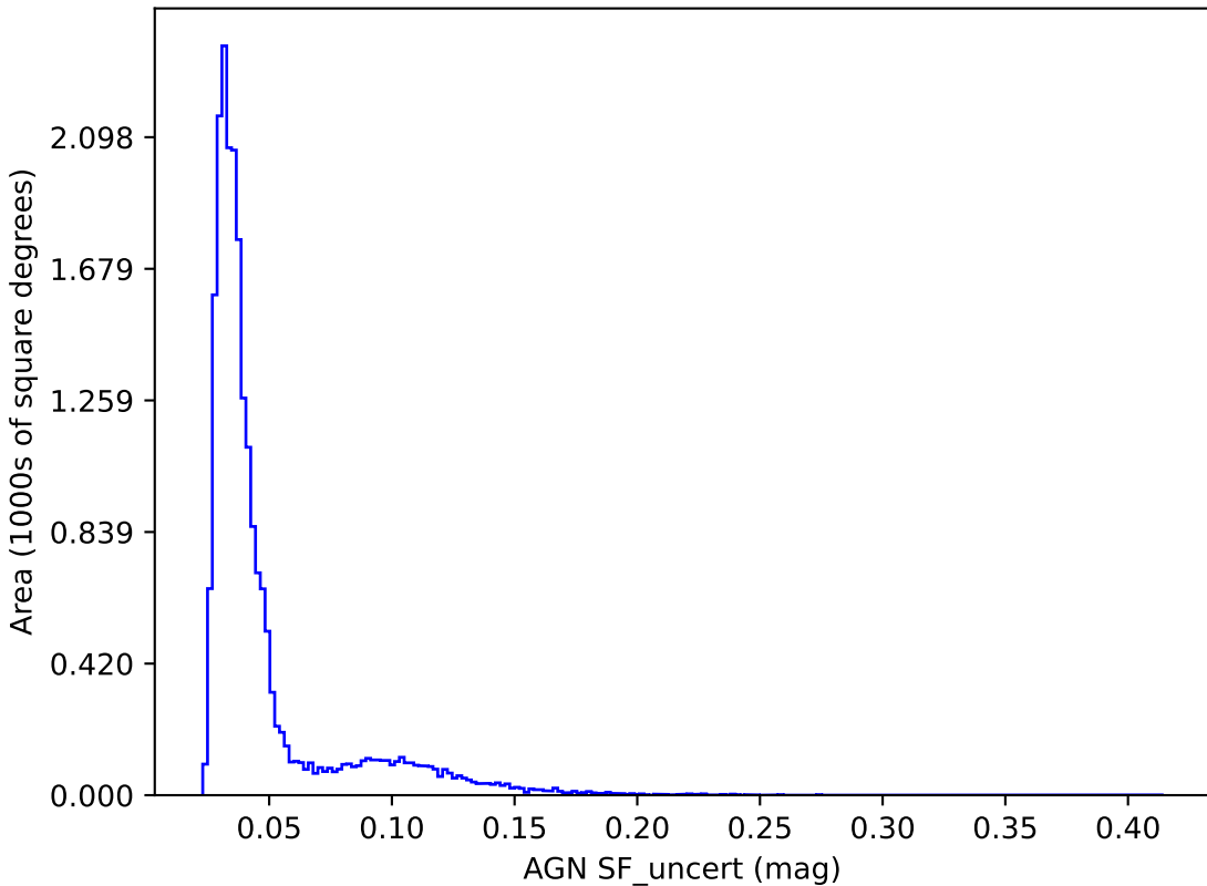
weather_cloudso4v3.4_10yrs y band: AGN SF_uncert
