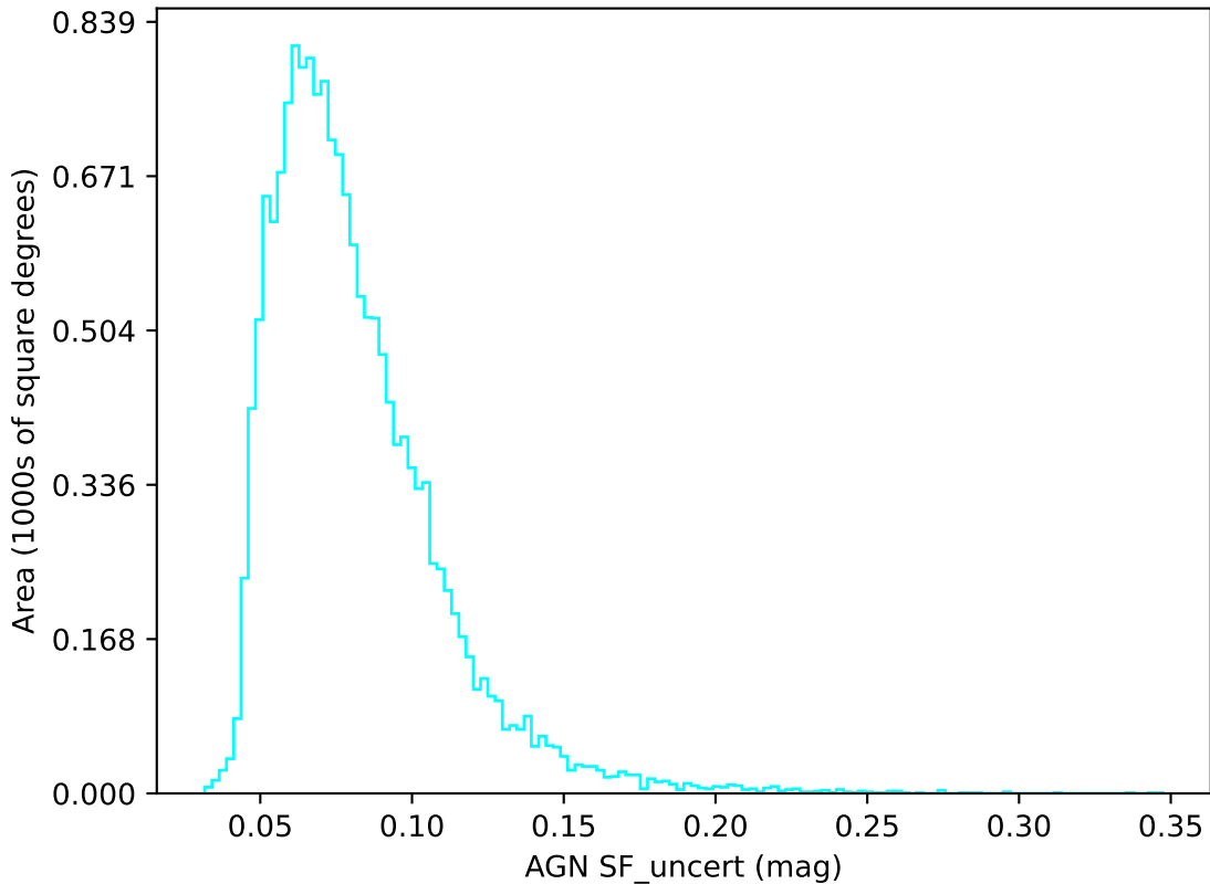
weather_cloudso4v3.4_10yrs u band: AGN SF_uncert
