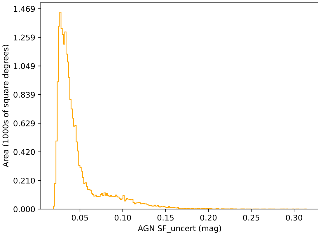
weather_cloudso4v3.4_10yrs r band: AGN SF_uncert
