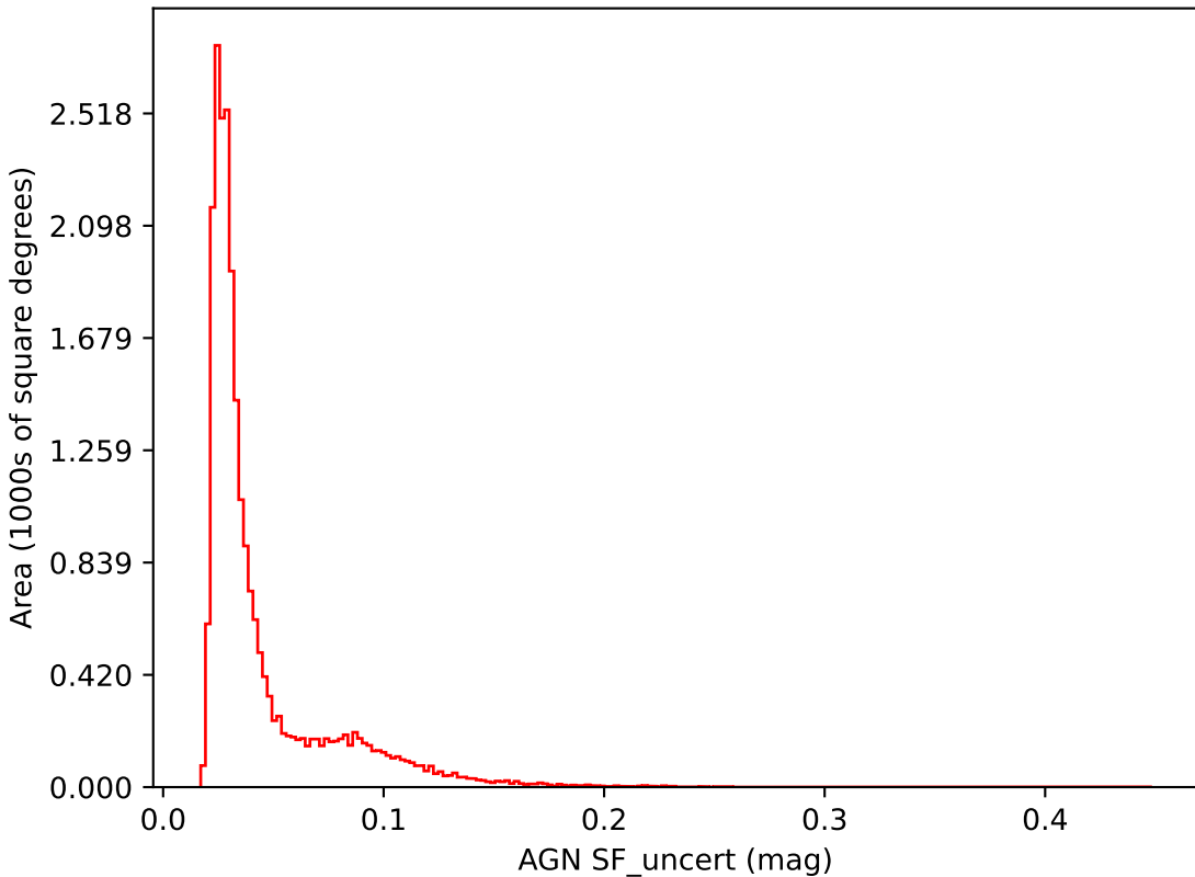
weather_cloudso4v3.4_10yrs i band: AGN SF_uncert
