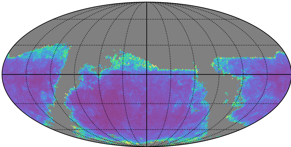
weather_cloudso4v3.4_10yrs g band: AGN SF_uncert
