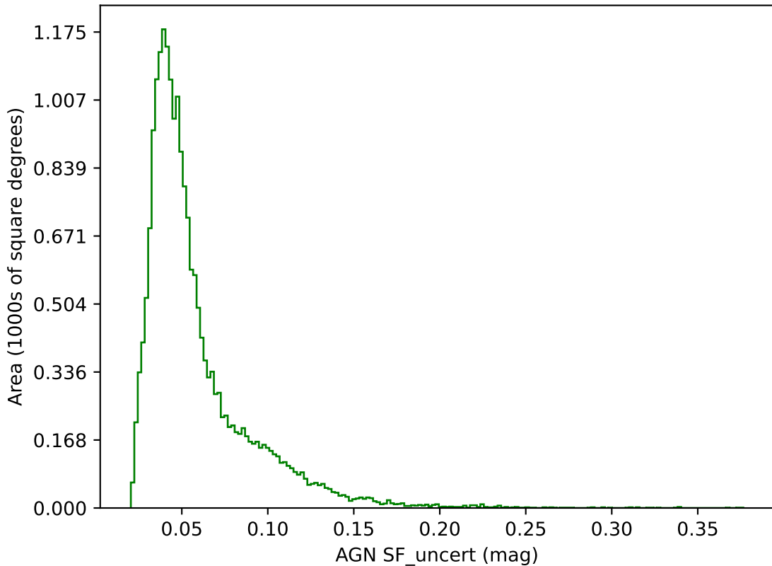
weather_cloudso4v3.4_10yrs g band: AGN SF_uncert
