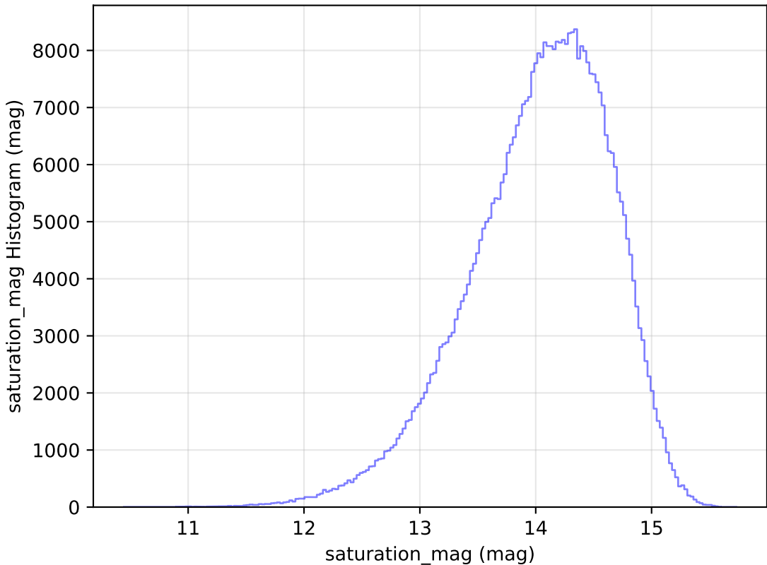
weather_cloudso4v3.4_10yrs WFD z band: saturation_mag Histogram
