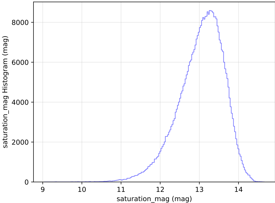
weather_cloudso4v3.4_10yrs WFD y band: saturation_mag Histogram
