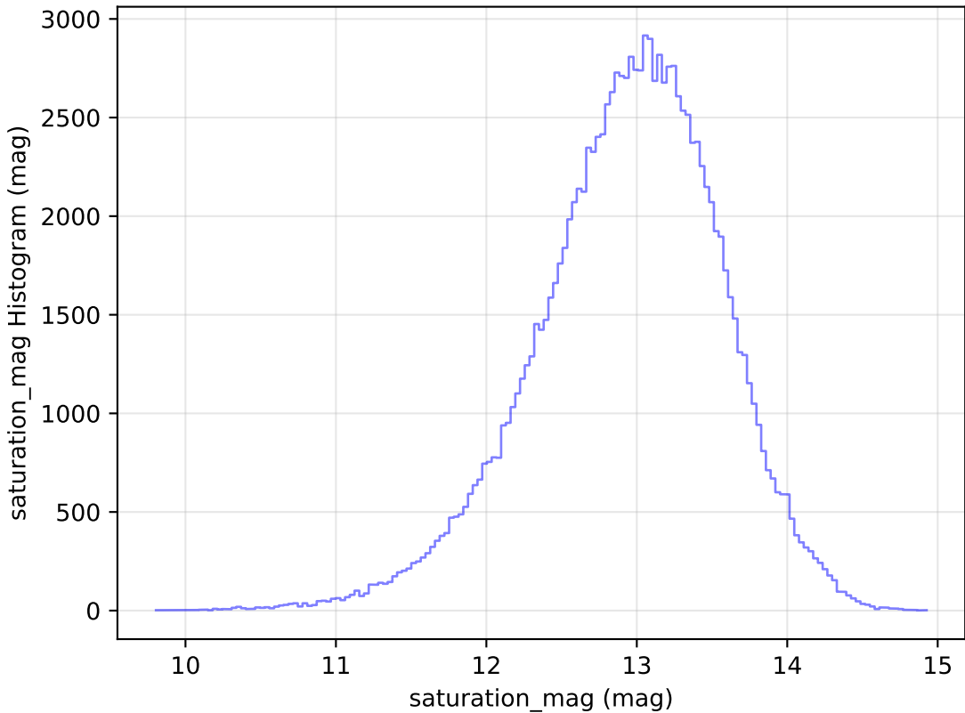
weather_cloudso4v3.4_10yrs WFD u band: saturation_mag Histogram
