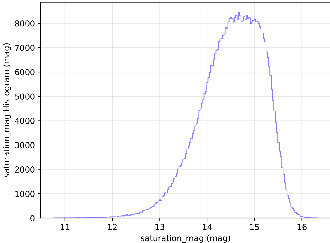
weather_cloudso4v3.4_10yrs WFD r band: saturation_mag Histogram
