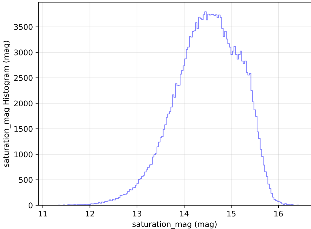
weather_cloudso4v3.4_10yrs WFD g band: saturation_mag Histogram
