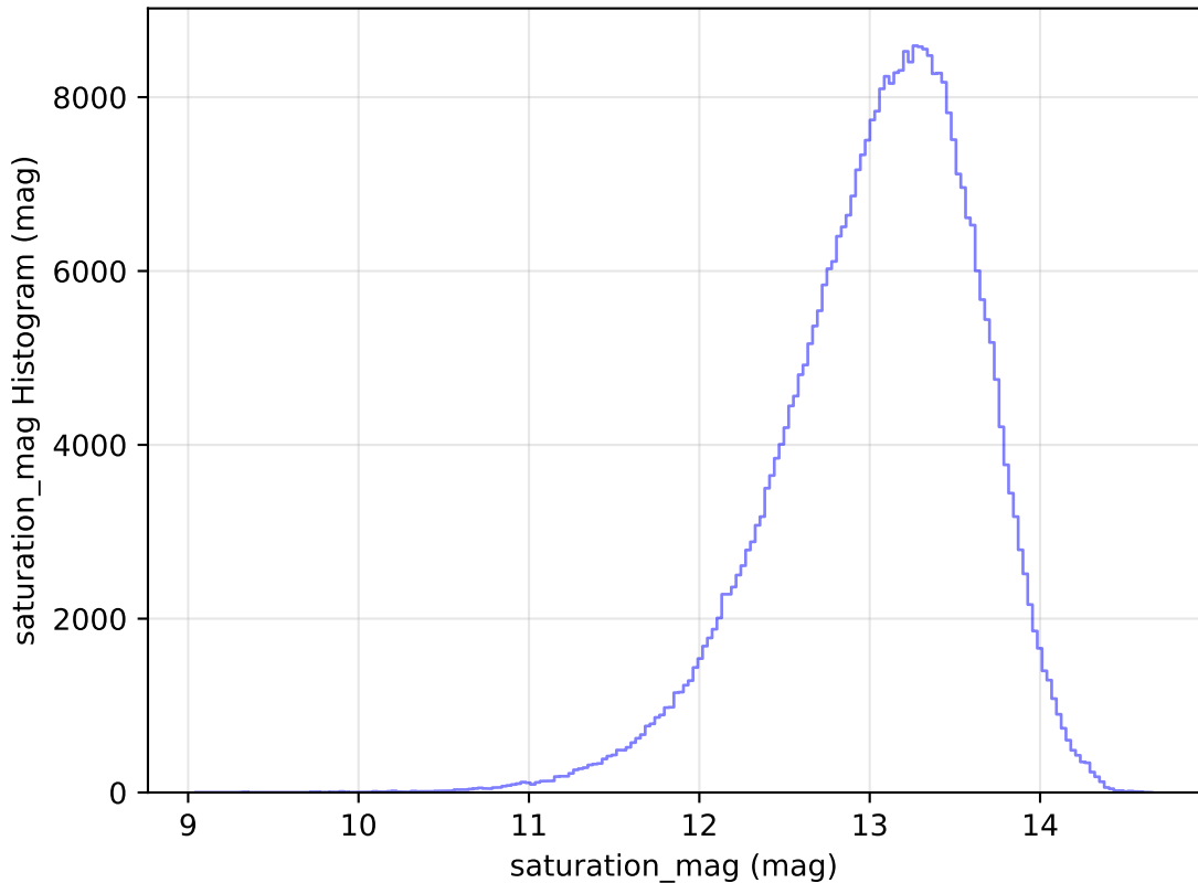
weather_cloudso4v3.4_10yrs All sky y band: saturation_mag Histogram
