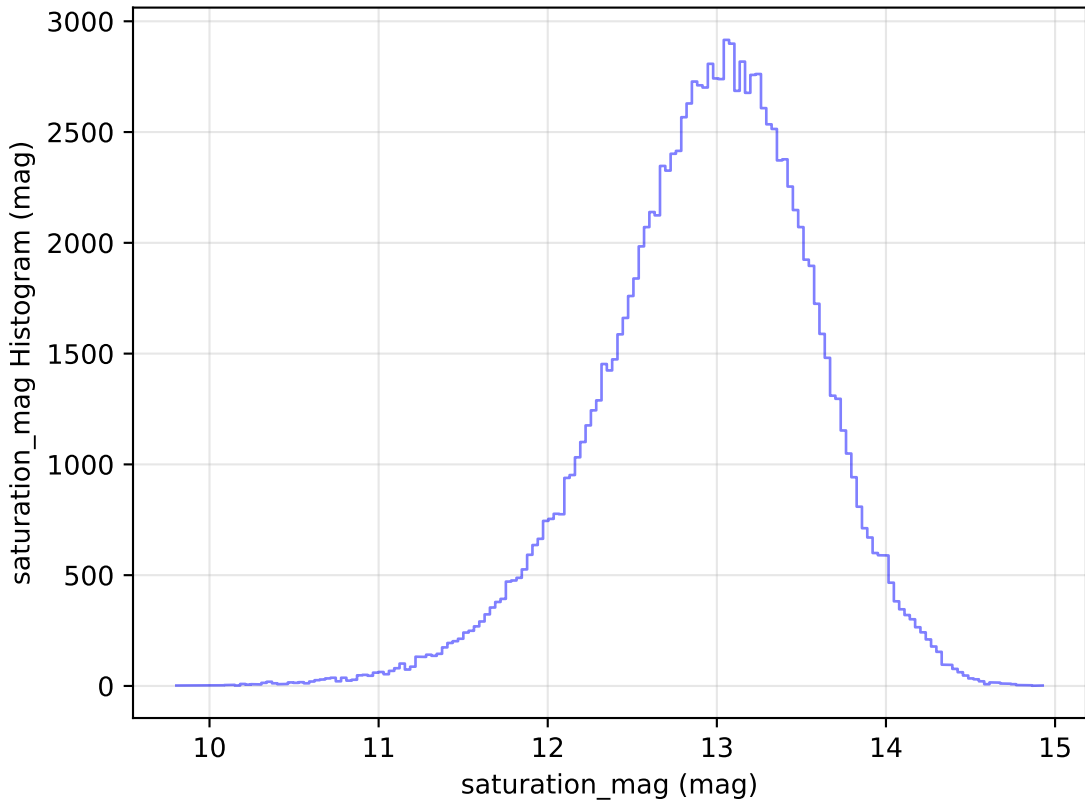
weather_cloudso4v3.4_10yrs All sky u band: saturation_mag Histogram
