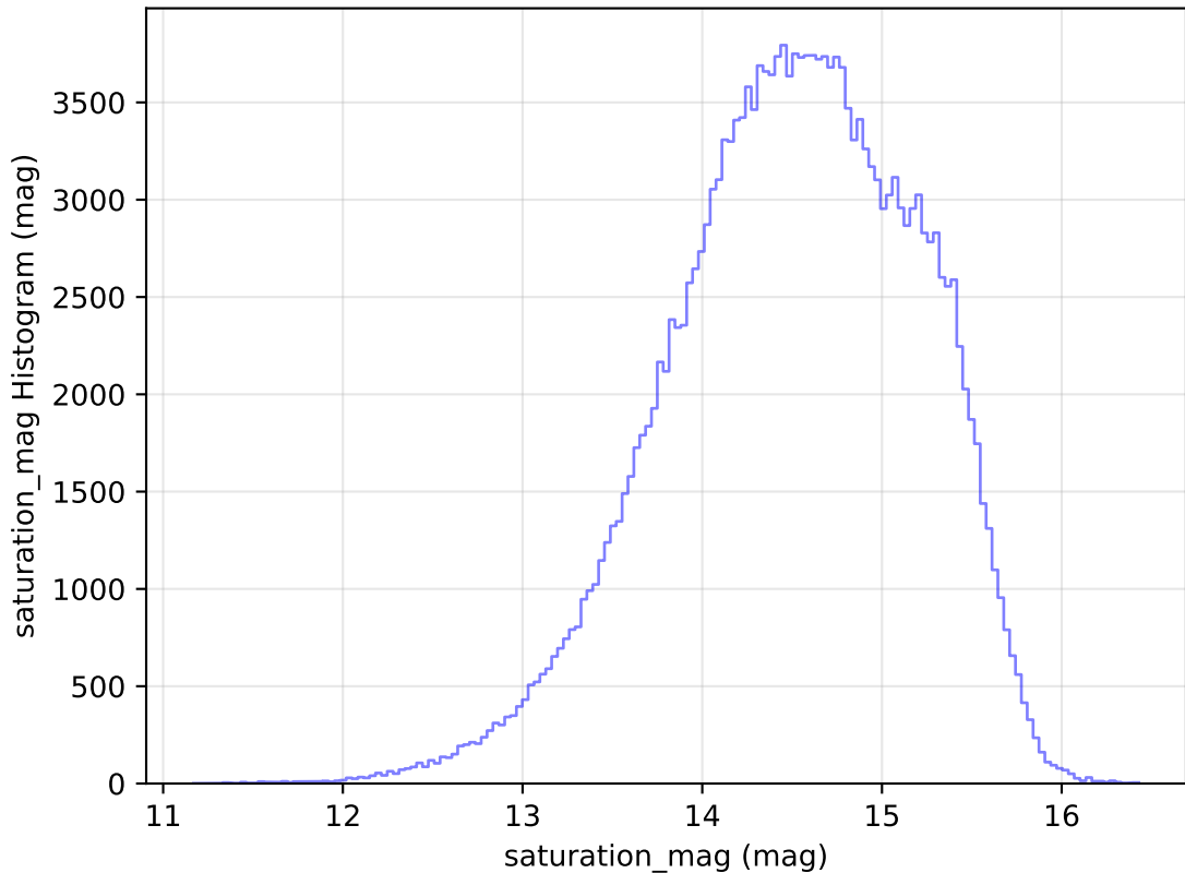
weather_cloudso4v3.4_10yrs All sky g band: saturation_mag Histogram
