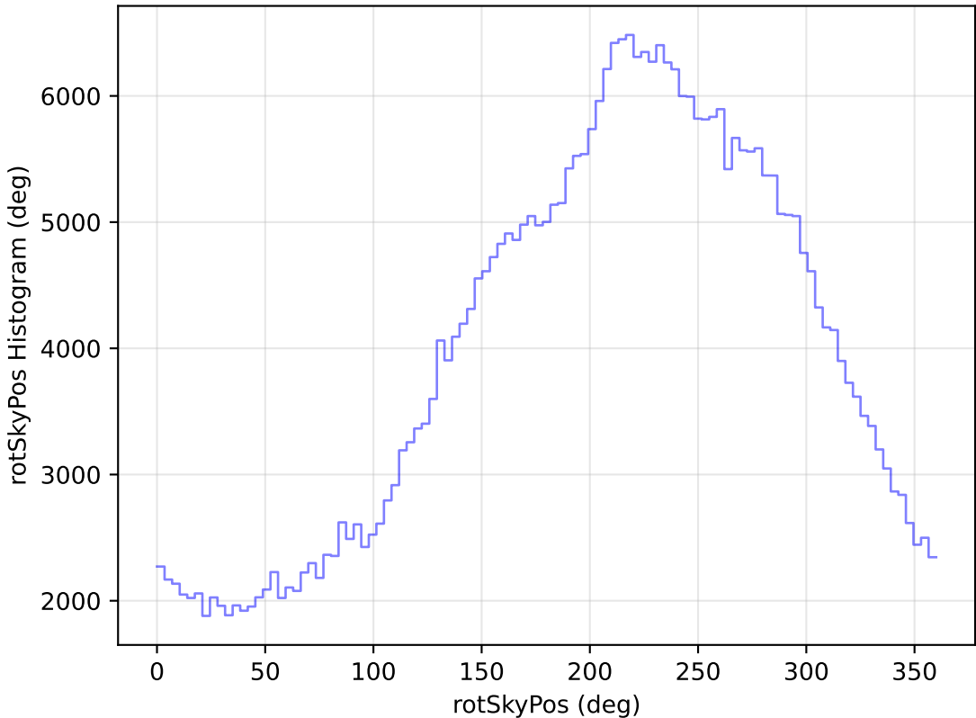
weather_cloudso4v3.4_10yrs WFD y band: rotSkyPos Histogram
