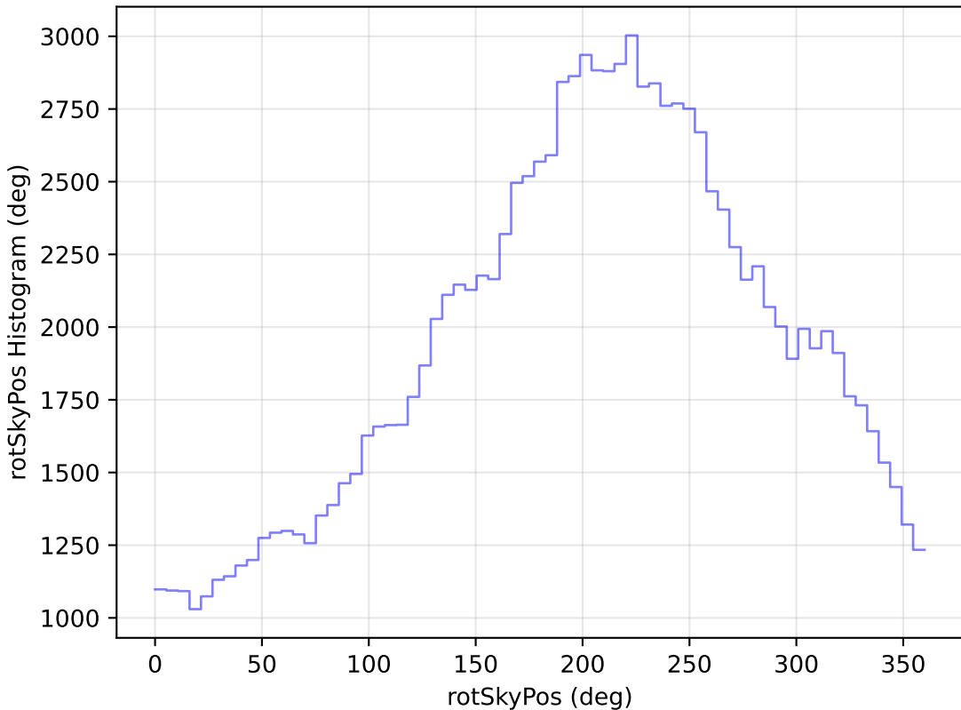
weather_cloudso4v3.4_10yrs WFD u band: rotSkyPos Histogram
