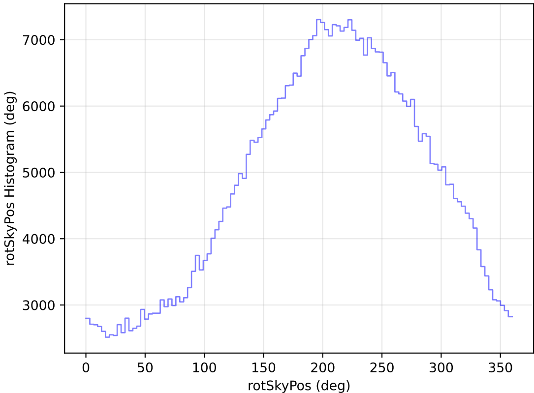
weather_cloudso4v3.4_10yrs WFD i band: rotSkyPos Histogram
