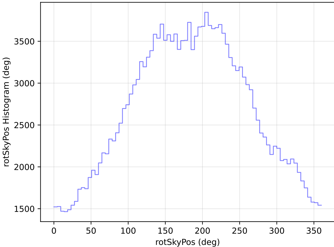
weather_cloudso4v3.4_10yrs WFD g band: rotSkyPos Histogram
