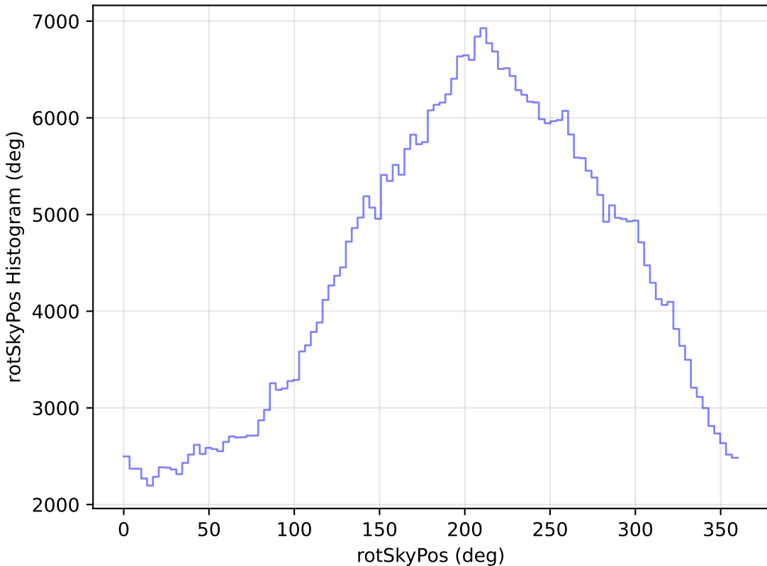
weather_cloudso4v3.4_10yrs All sky z band: rotSkyPos Histogram
