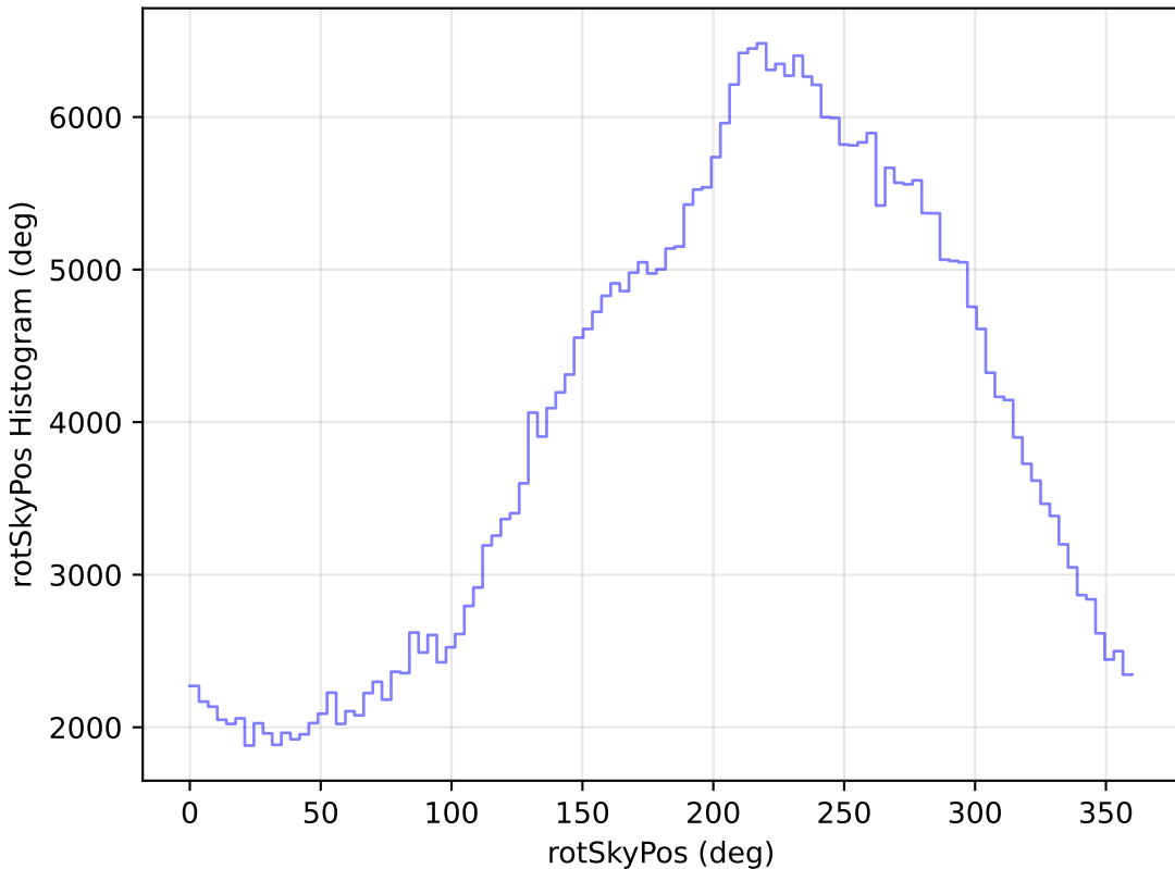
weather_cloudso4v3.4_10yrs All sky y band: rotSkyPos Histogram
