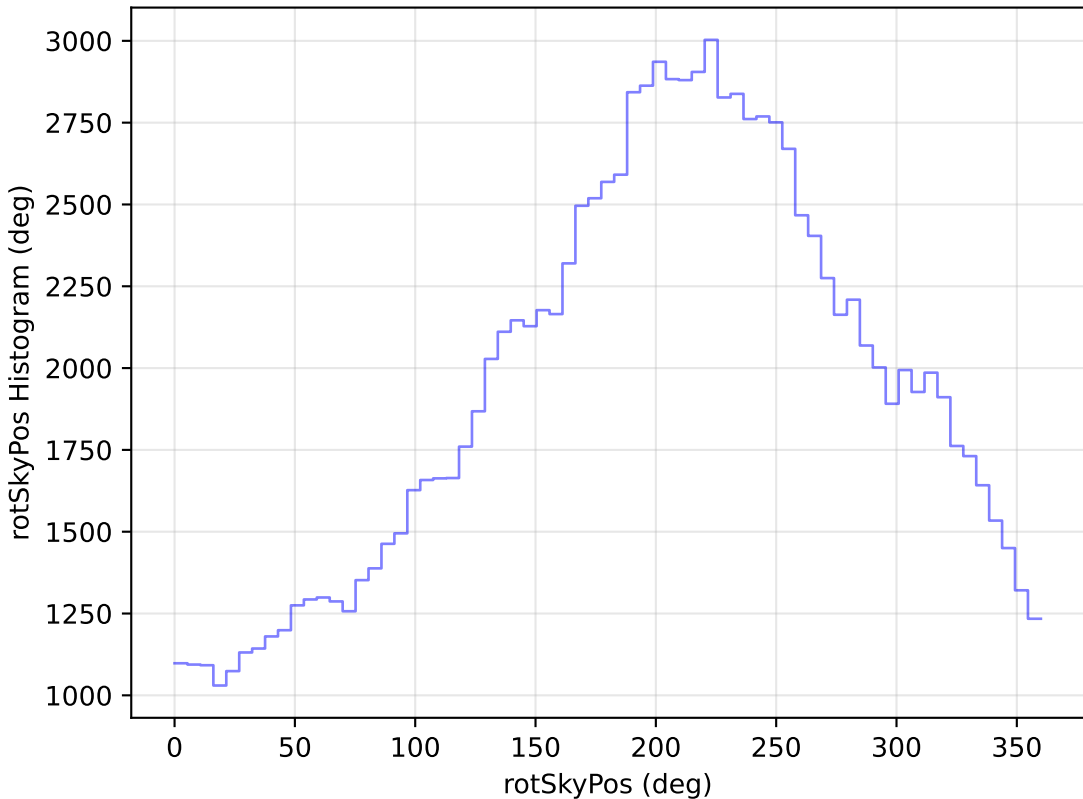
weather_cloudso4v3.4_10yrs All sky u band: rotSkyPos Histogram
