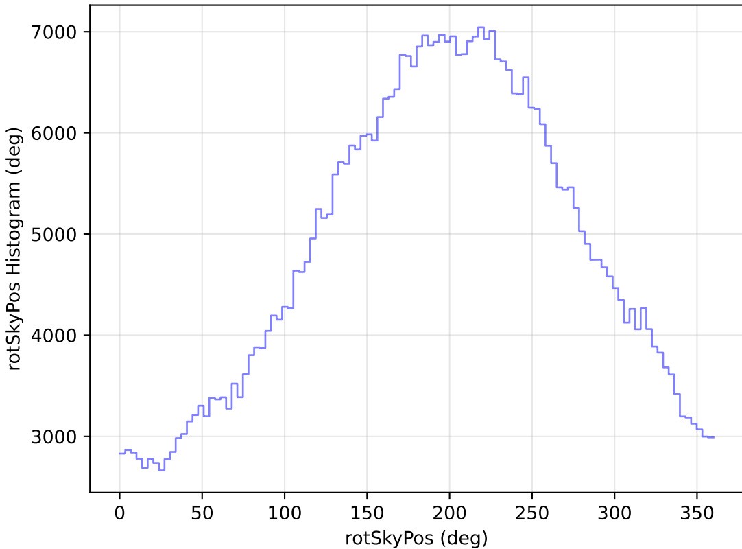
weather_cloudso4v3.4_10yrs All sky r band: rotSkyPos Histogram
