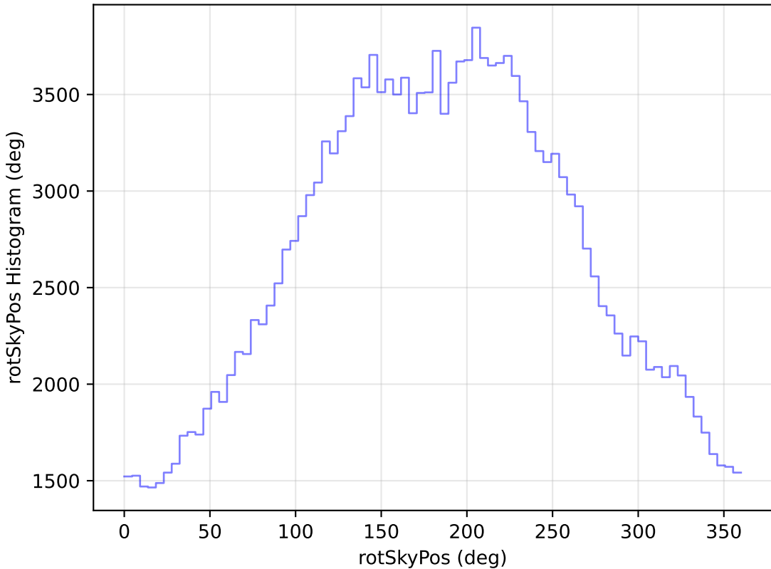
weather_cloudso4v3.4_10yrs All sky g band: rotSkyPos Histogram
