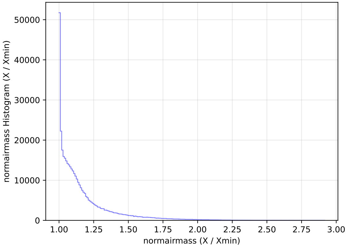
weather_cloudso4v3.4_10yrs WFD y band: normairmass Histogram
