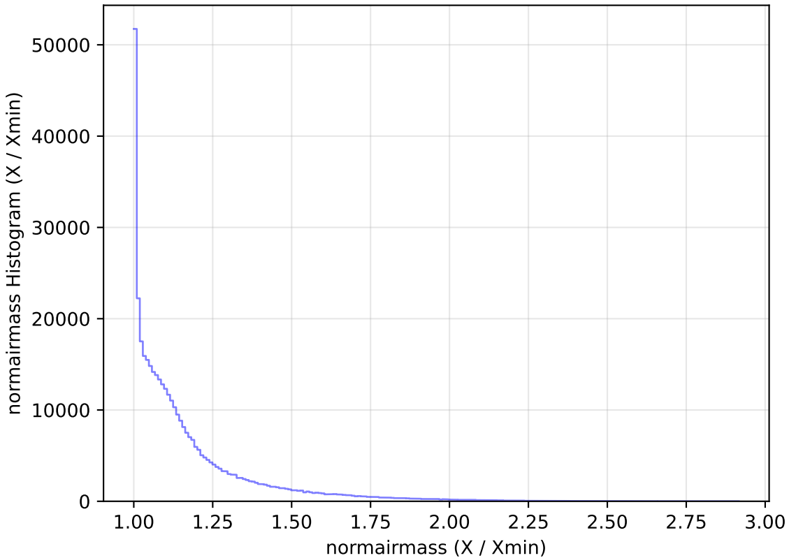
weather_cloudso4v3.4_10yrs All sky y band: normairmass Histogram
