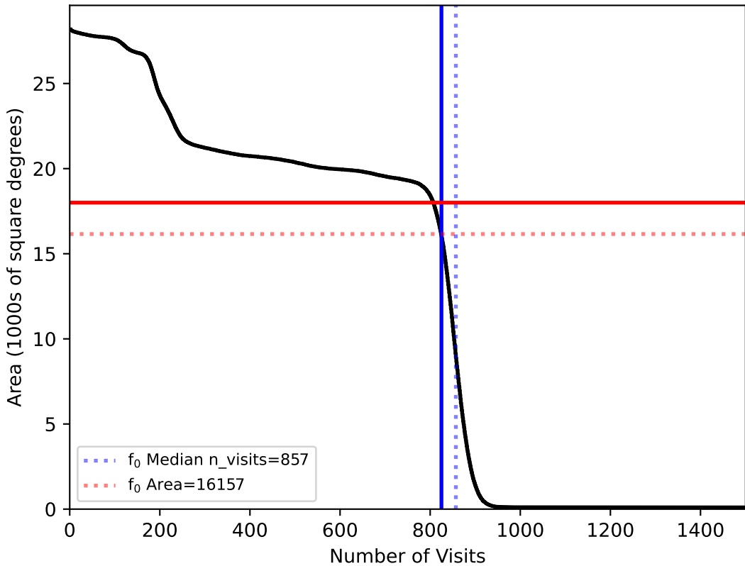
weather_cloudso4v3.4_10yrs All sky: f0
