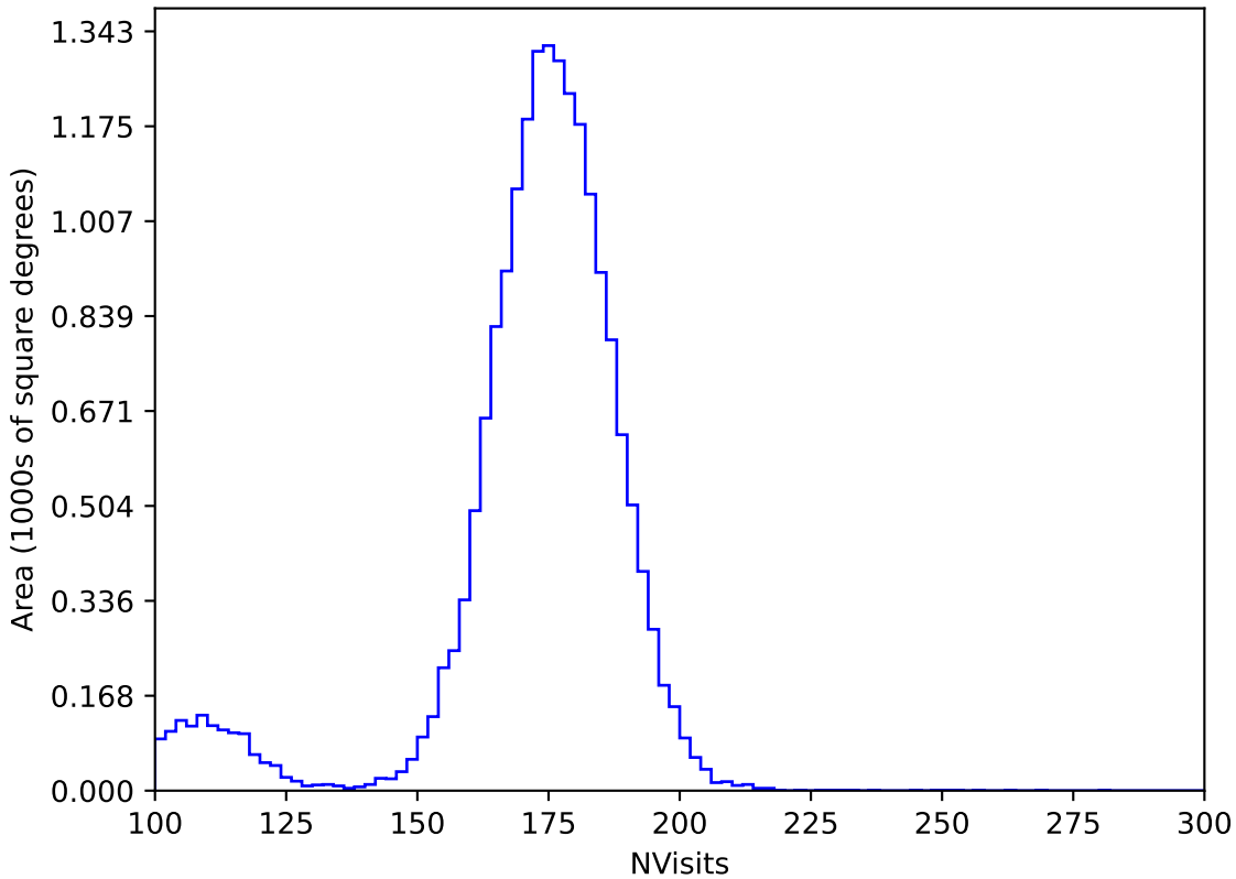
weather_cloudso4v3.4_10yrs WFD y band: NVisits
