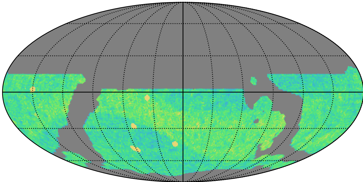
weather_cloudso4v3.4_10yrs WFD i band: NVisits
